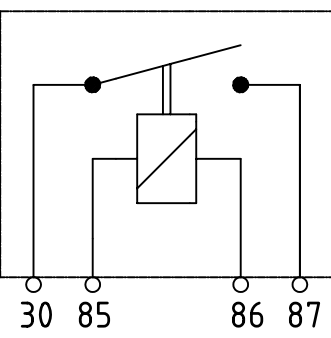
Schaltbild / wiring diagram
