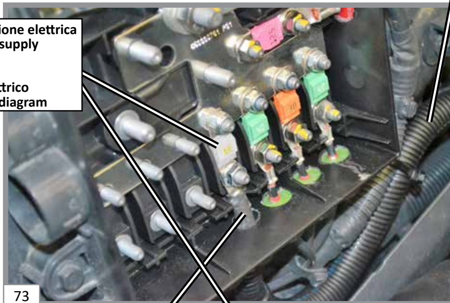
Cablaggio - Alimentazione elettrica Wiring - Power supply
