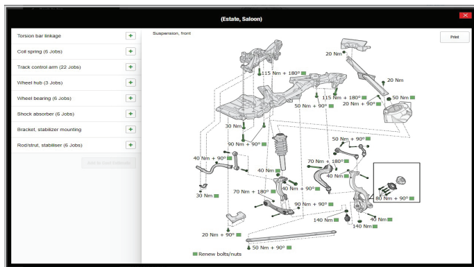
Tekniset piirroksset kiristysmomenteilla
