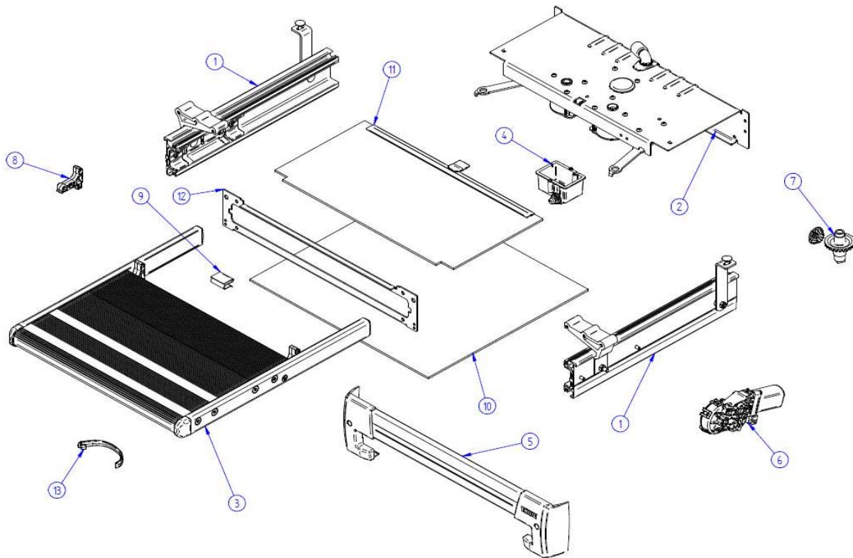
THULE Slide Out V19 12V DU/JU/BO
