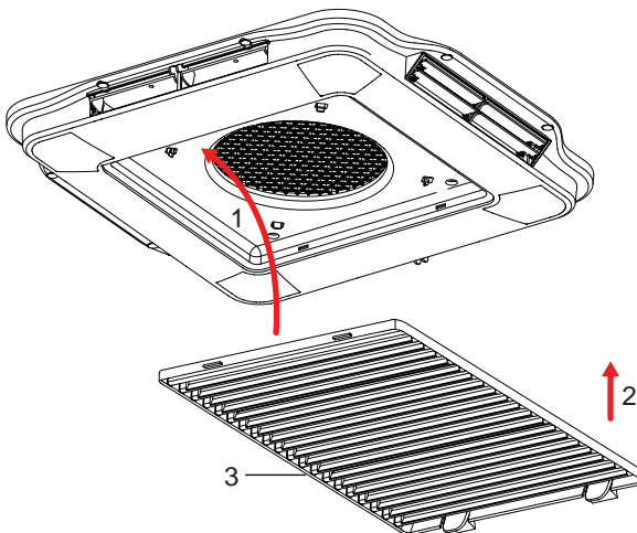
Kuva 20: Ilmansuodattimen asennus
