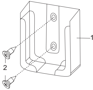
Kuva 21: Kauko-ohjaimen pidike
