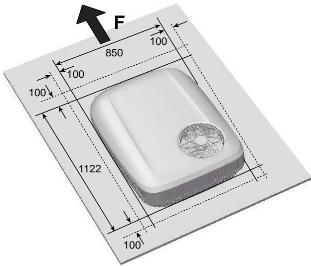
Kuva 01: Ulkoyksikön asennussuunta
