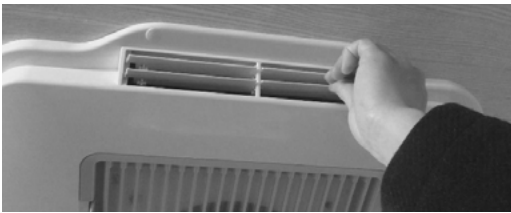
Kuva 42: Ilmanpoistokohdan (1) säätäminen
