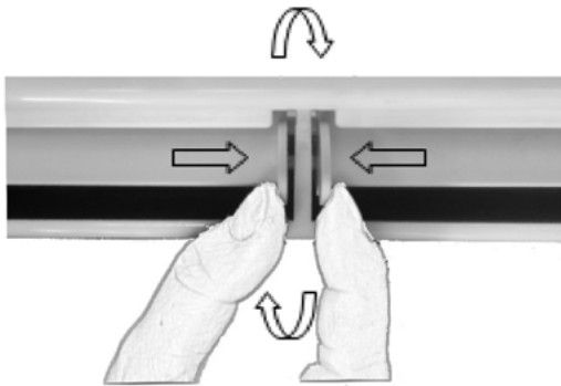
Kuva 43: Ilmanpoistokohdan (2) säätäminen
