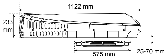
Kuva 03: Asennusmitat (kuva sivulta)
