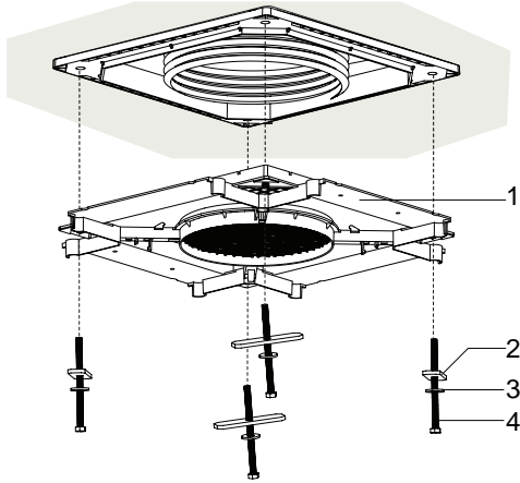
Kuva 13: M8-pulttien asennus
