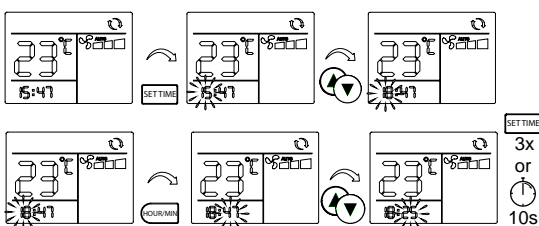
Kuva 33: Kellon asetus
