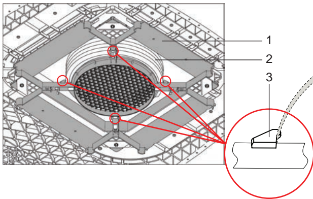
Kuva 14: Ilmanottokanavan liittäminen
