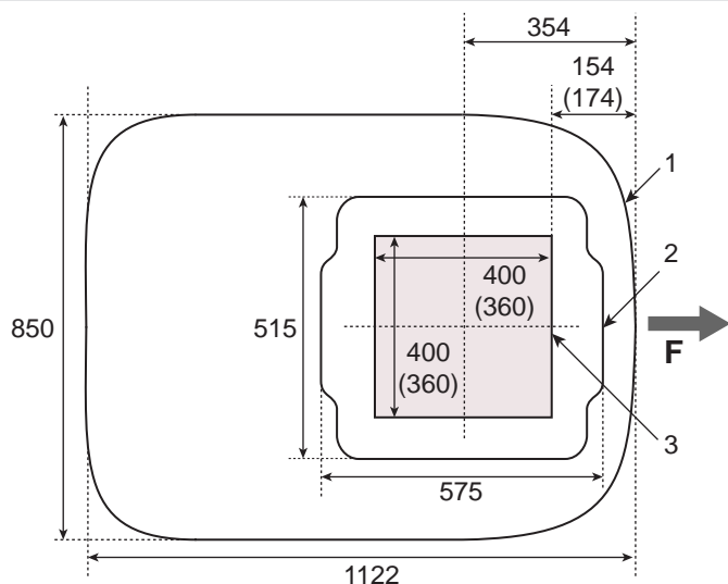
Kuva 02: Asennustoimenpiteet (näkökulma ylhäältä/alhaalta)
